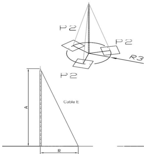
Modelo de torre arriostrada 180 Altura 5 - 7'5 - 10 metros
