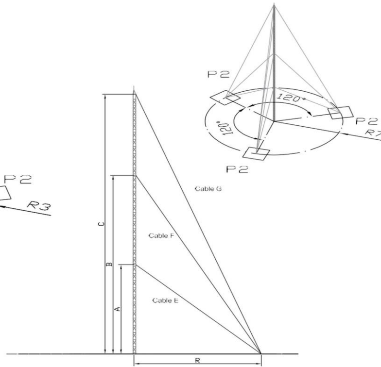
Torre arriostrada modelo 180 Altura 12'5 - 15 - 17'5 metros
